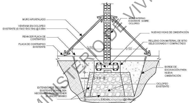
Figura A. 2-9 Nueva viga de cimentación en concreto reforzado para muros perimetrales nuevos junto a muros compartidos.
