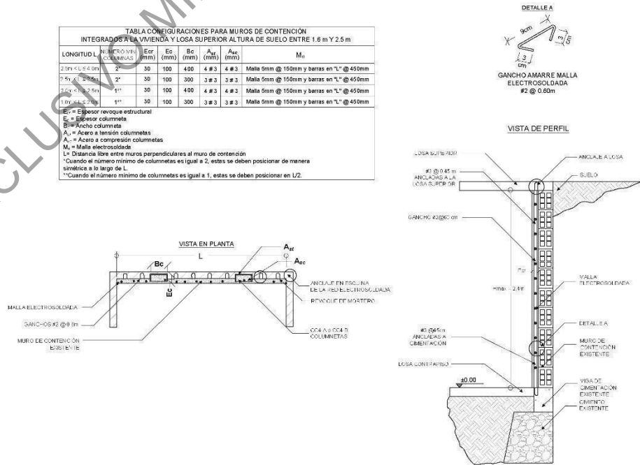
Figura A.2 -2 Refuerzo de muro de contención integrado a la vivienda con losa superior existente – Altura del suelo entre 1.8m y 2.5m.
