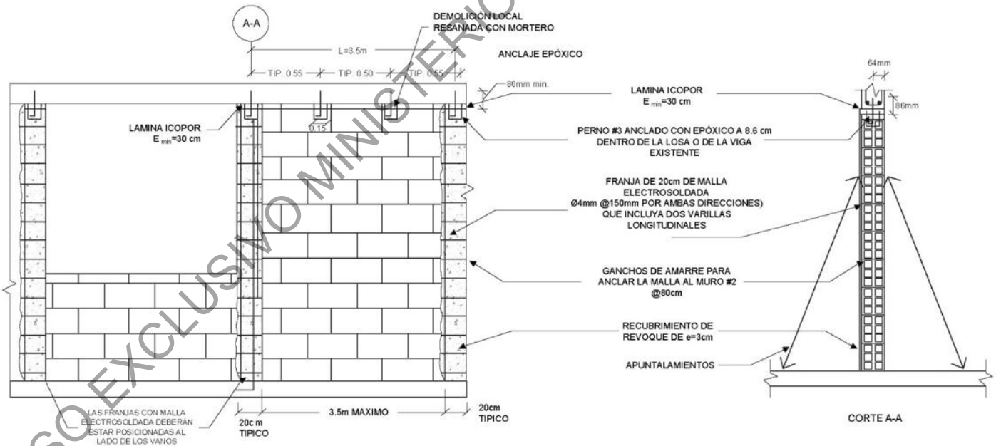
Figura A. 2-15 Dilatación de muros existentes.
