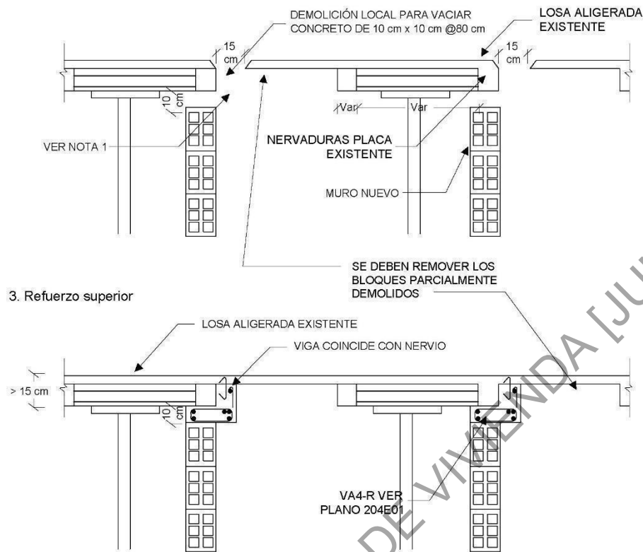
Figura A. 2 -20 Conexión de muro nuevo a losa existente con nervios. Muro coincidente con los nervios.
