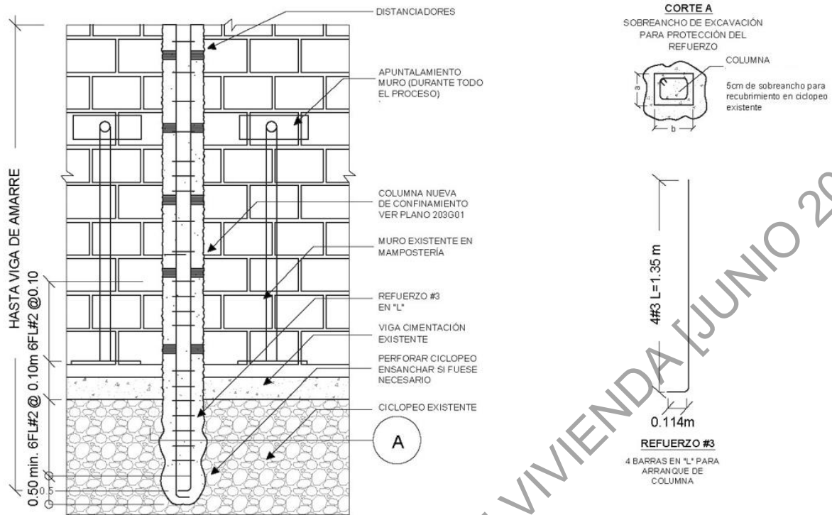
Figura A. 2-12 Anclaje de nueva columna de confinamiento a cimentación existente.
