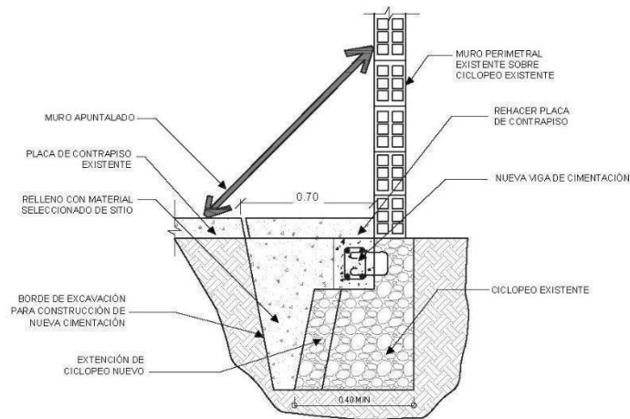
Figura A. 2-8 Nueva viga de cimentación en concreto reforzado para muros internos sobre concreto ciclópeo existente.
