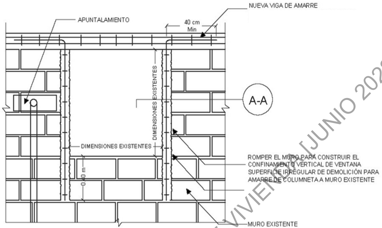
Figura A. 2-14 Refuerzo de vanos existentes.
