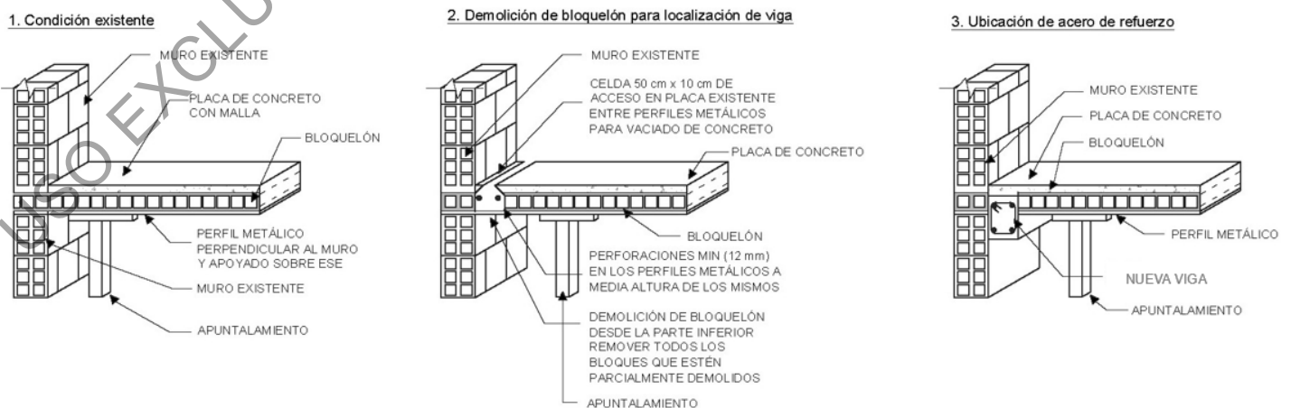
Figura A. 2 -21 Construcción de nueva viga para dar rigidez al diafragma. Viga perpendicular a los perfiles metálicos.
