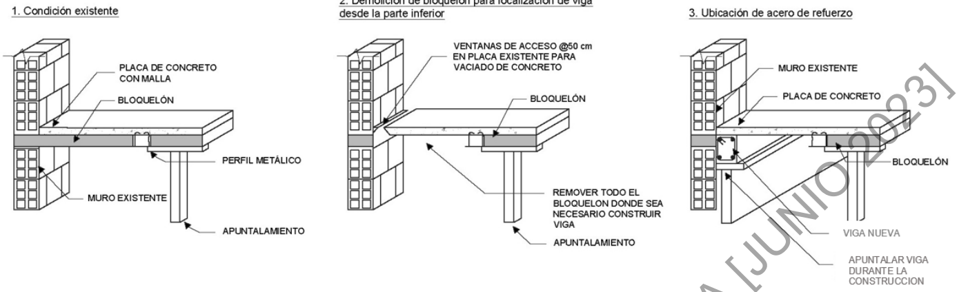
Figura A. 2 -22 Construcción de nueva viga para dar rigidez al diafragma. Viga paralela a los perfiles metálicos.
