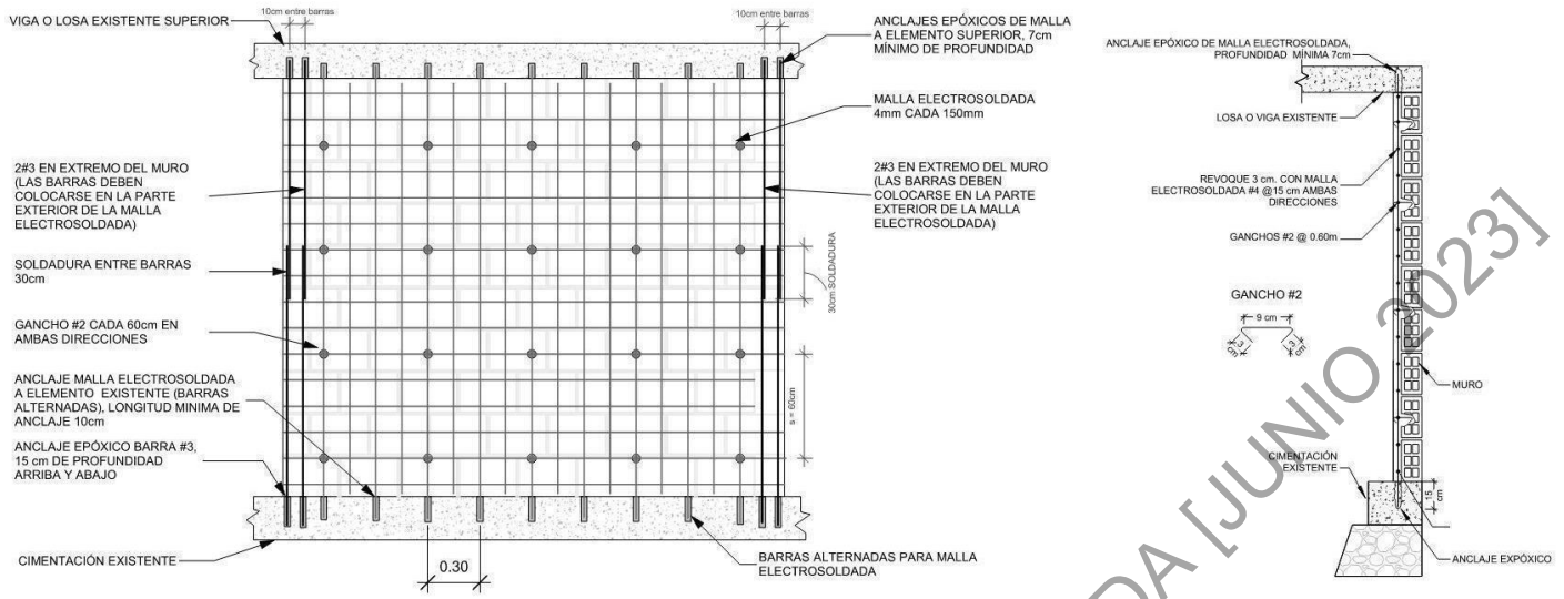
Figura A. 2-16 Refuerzo de muro existente con de revoque con malla.
