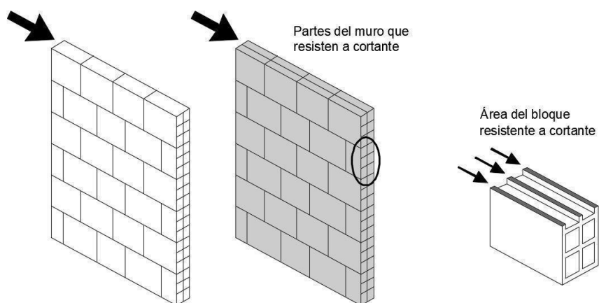
Figura 5.10.1-1 Área del bloque resistente a corte
