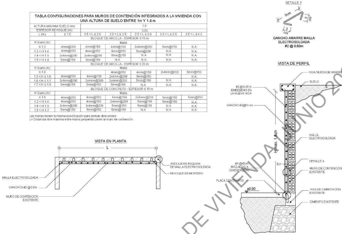
Figura A. 2-4 Refuerzo de muro de contención integrado a la vivienda con nueva losa o viga de amarre superior - Altura del suelo entre 1.8m y 2.5m
