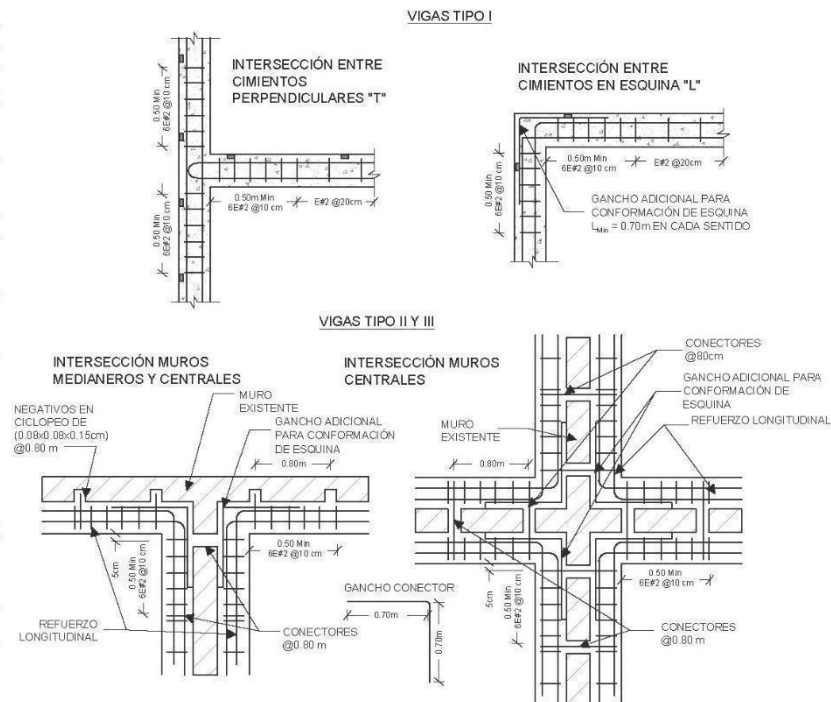
Figura A. 2-6 Despiece de nuevas vigas de cimentación para refuerzo de sistemas existentes.
