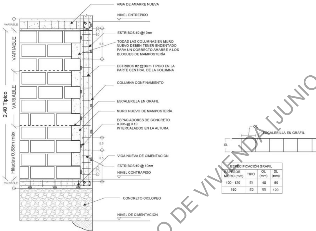
Figura A. 2-10 Sección típica de nuevo muro.
