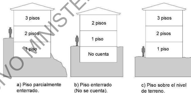
Figura 6.3.3-1 Esquema para definir número de niveles
