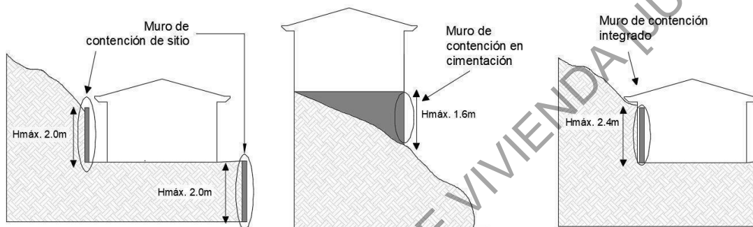
Figura 6.2.3-1 Tipologías de muro de contención
