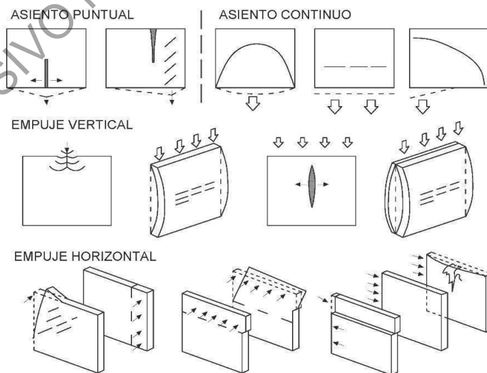
Figura 6.4.1-1 Tipos de fisuras
