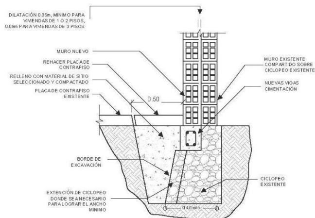
Figura A. 2-9 Nueva viga de cimentación en concreto reforzado para muros perimetrales nuevos junto a muros compartidos.
