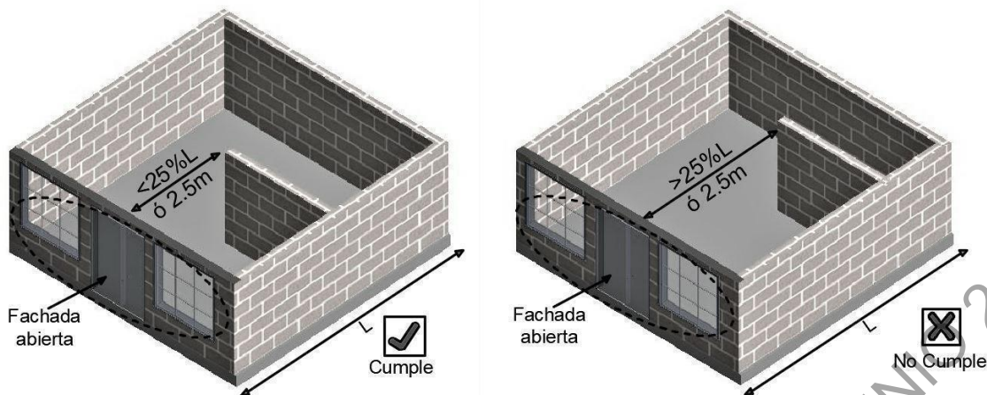
Figura 7.4.2-1 Chequeo parámetros para torsión
