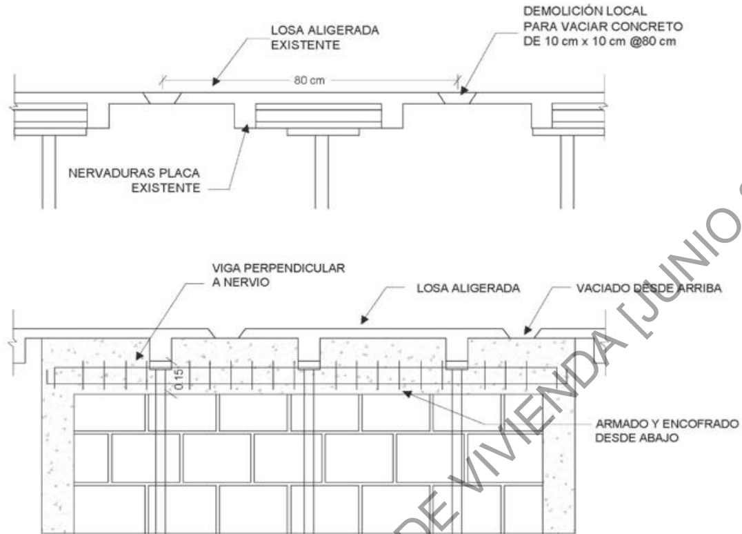
Figura A. 2-18 Conexión de muro nuevo a losa existente con nervios. Muro perpendicular a los nervios.
