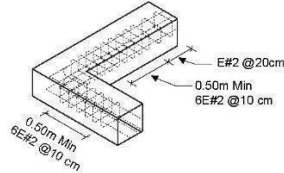
UNIÓN DE VIGA DE AMARRE EN ESQUINA
